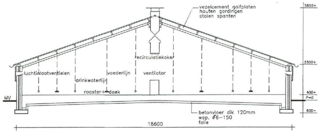
dwarsdoorsnede
