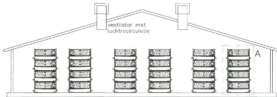
dwarsdoorsnede
