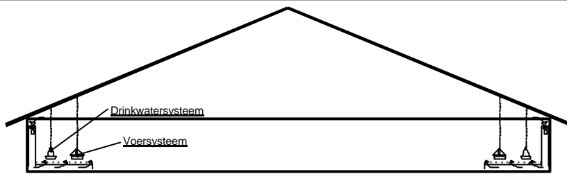
Doorsnede variant A
