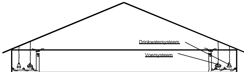
Doorsnede variant B
