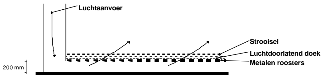
Detail verhoogde vloer
