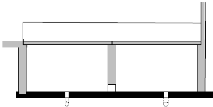
Doorsnede A - A (diepe mestkanalen, eventueel voorzien van riolering)
