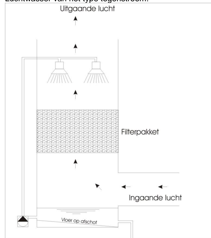
Luchtwasser van het type tegenstroom:
