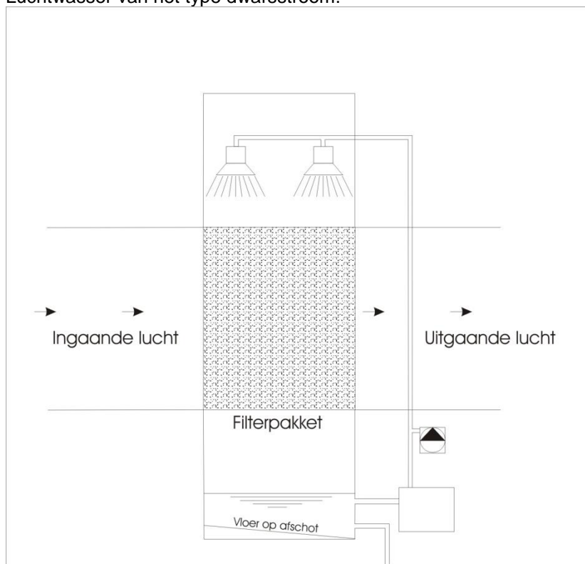
Luchtwasser van het type dwarsstroom:
