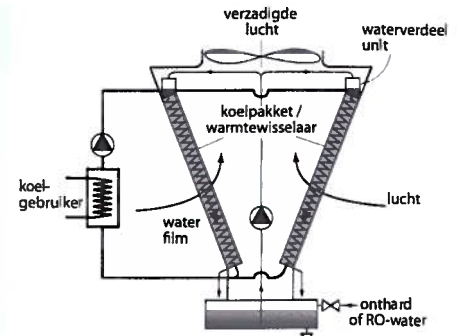
Hybride koeler met recirculatie filmend
