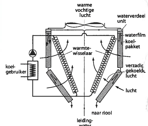
Adiabatische koeler zonder recirculatie (filmend)
